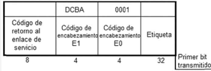
FIGURA 36.- Mensaje de retorno al enlace de servicio.
