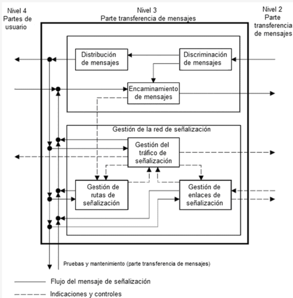
FIGURA 24.- Funciones de la red de señalización.
