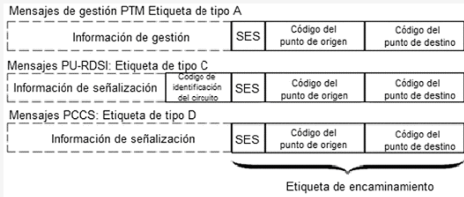
FIGURA 10.- Tipos de etiqueta de mensajes de SS7.
