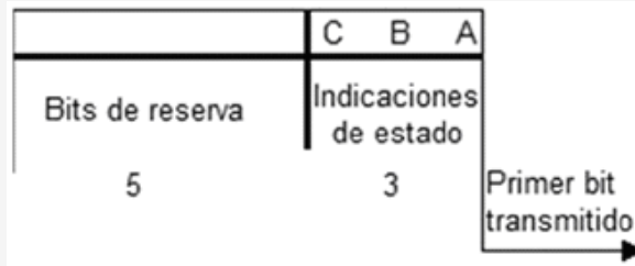
FIGURA 22.- Formato del campo de estado.
