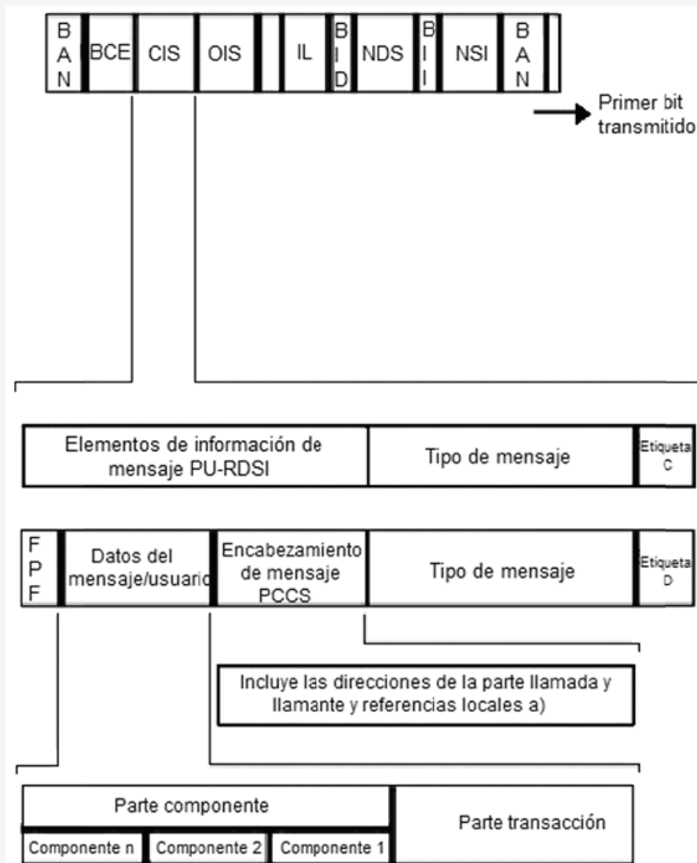
FIGURA 10.- Tipos de etiqueta de mensajes de SS7.
