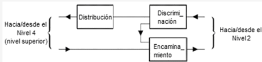
FIGURA 25.- Encaminamiento, discriminación y distribución de mensajes.
