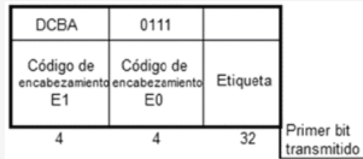
FIGURA 41.- Mensaje de reanudación de tráfico autorizada.
