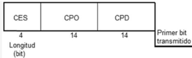
FIGURA 34.- Estructura normalizada de la etiqueta.
