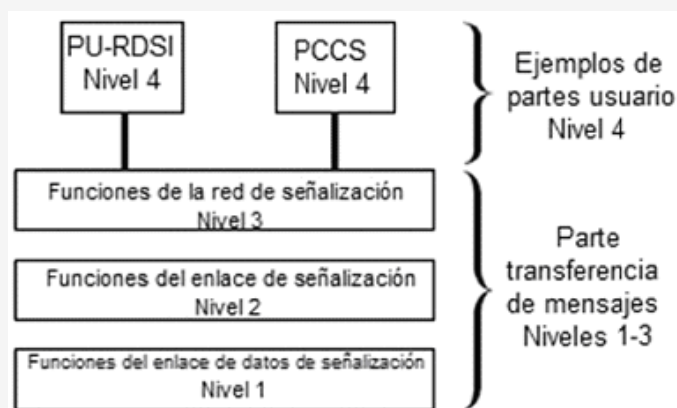
FIGURA 3.- Niveles funcionales del SS7.
