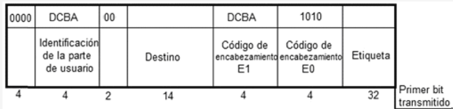
FIGURA 42-C.- Mensaje de parte de usuario indisponible.
