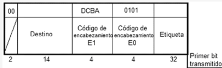
FIGURA 40.- Mensaje de prueba de conjunto de rutas de señalización.
