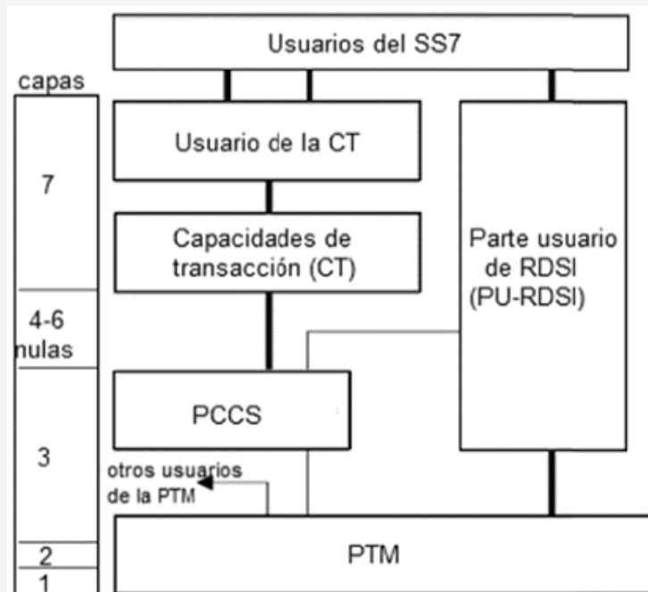
FIGURA 2.- Arquitectura del sistema de señalización N.º 7.
