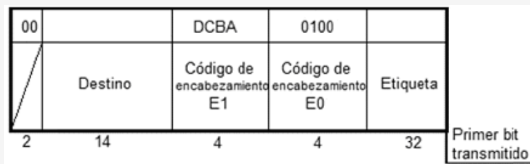
FIGURA 39.- Mensaje de transferencia autorizada.
