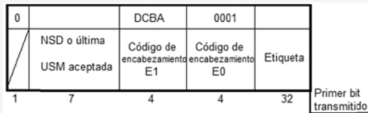
FIGURA 35.- Mensaje de paso a enlace de reserva.
